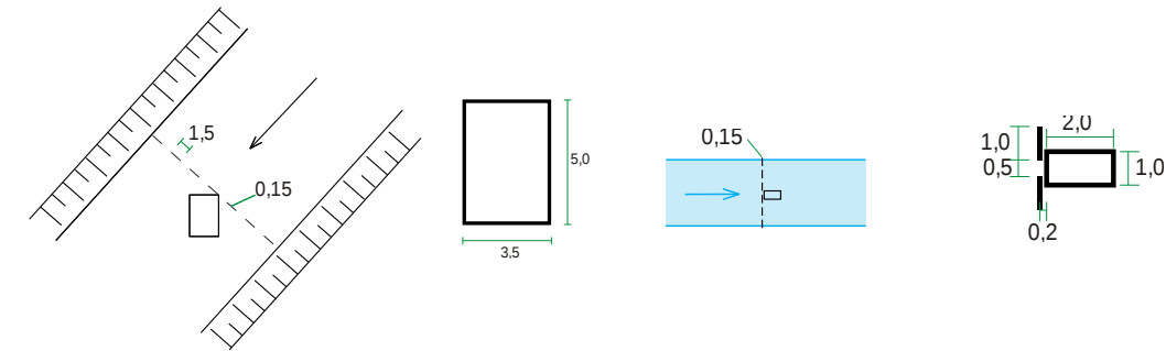
5.1.20. Skela za vozila
