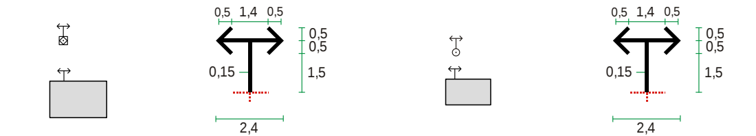
4.11.16. Antena na nosaču na zgradi
