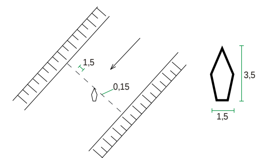
5.1.21. Skela za pješake
