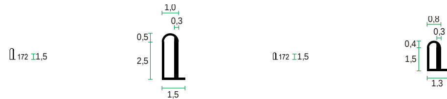
5.1.22. Kilometarska oznaka uz prometnicu
